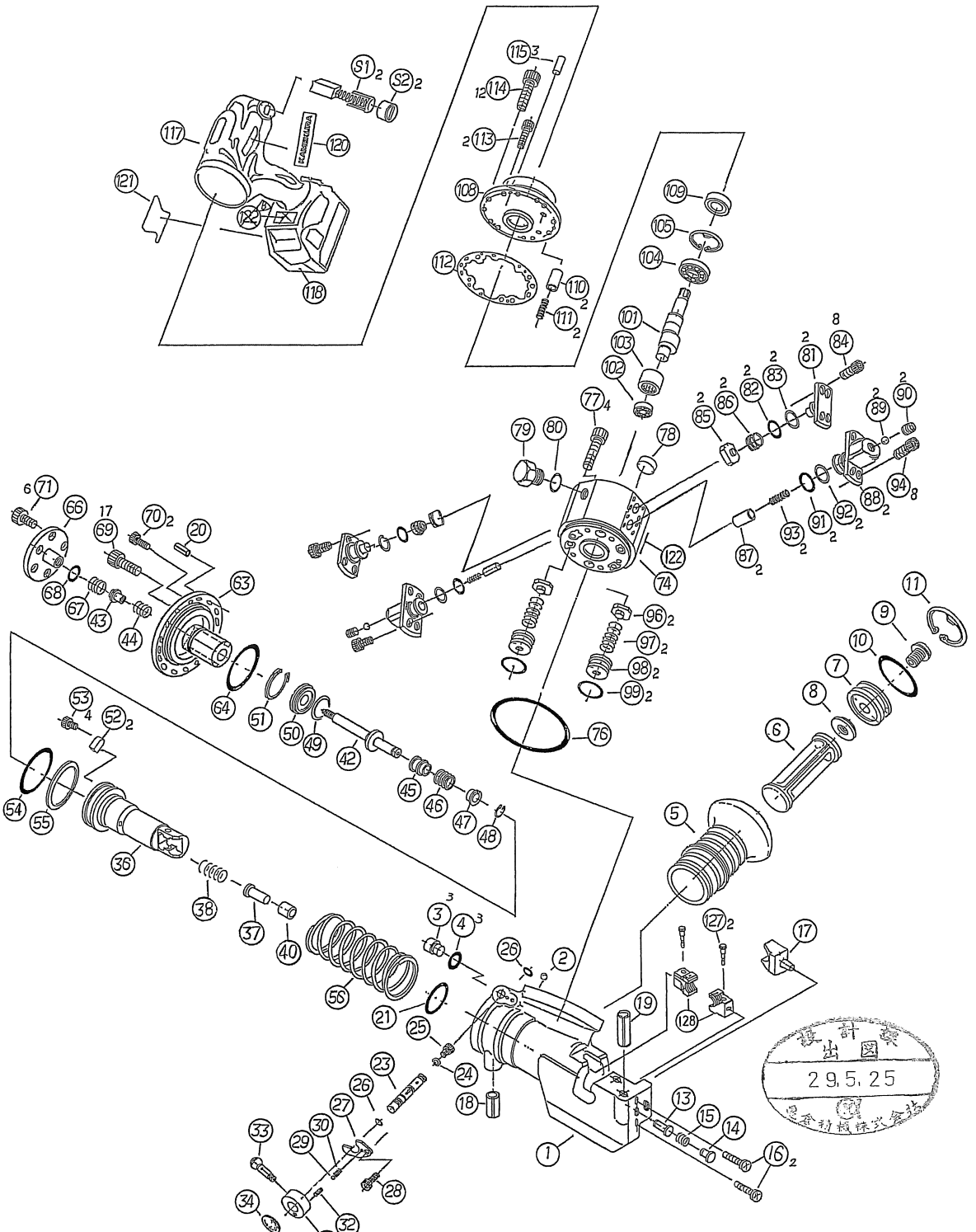
DW-408B コードレスハートカッター 分解図 (DW-B002)
